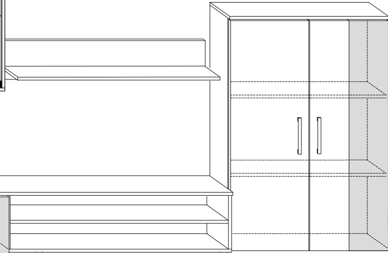
H-19 D-20 L-100 STE-02 PÓŁKI ( 2 SZT. )
