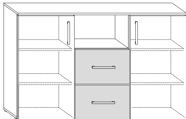
H-88 D-42 L-135 STE-01 KOMODA
