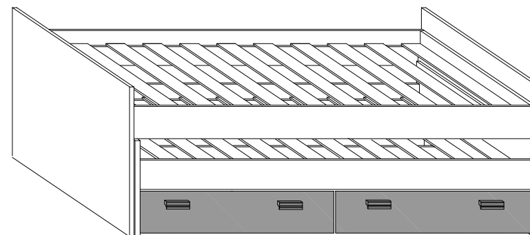
H-77 D-98 L-212 KIT-07 ŁÓŻKO PODWÓJNE
