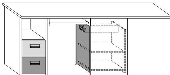
H-79 D-55 L-191 KIT-02 BIURKO NAROŻNE
