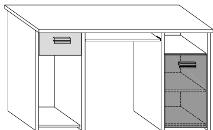
H-75 D-55 L-125 KIT-01 BIURKO
