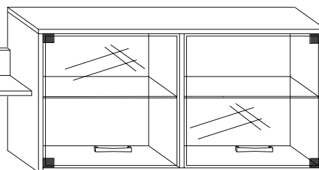
H-48 D-32 L-96 MAG-07 SZAFKA WISZĄCA POZIOMA
