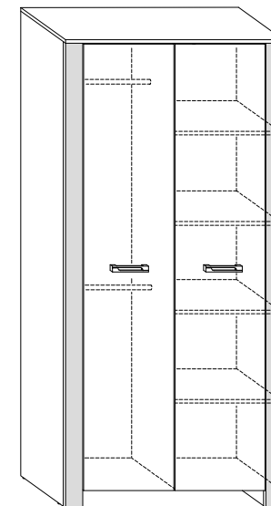
H-195 D-58 L-90 HUG-10 SZAFKA
