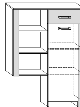
H-128 D-40 L-90 HUG-06 REGAŁ NISKI
