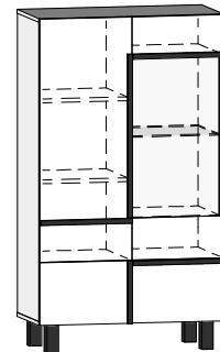
LAR-12 WITRYNA 1D1S L-80 H-142 D-42
