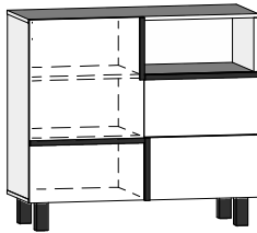
LAR-01 KOMODA 1D2S L-100 H-90 D-42
