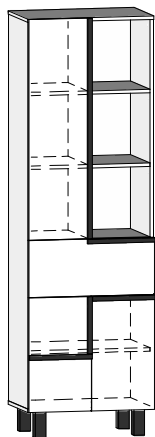
LAR-07 REGAŁ 3D1S L-60 H-195 D-42
