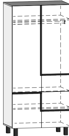
LAR-10 SZAFKA 4D L-90 H-195 D-59
