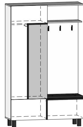
LAR-06 PRZEDPOKÓJ 3D L-120 H-195 D-42
