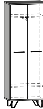
BOS-14 SZAFKA 2D L-60 H-170 D-39 * montaż z wieszakiem
