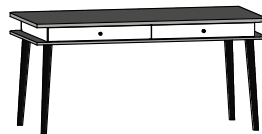
DOL-19 Stół L-160 H-76 D-82
