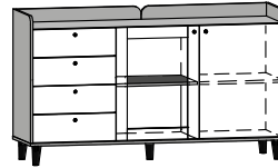
DOL-04 Komoda 1D4SW L-160 H-91 D-46
