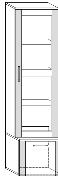
NOT-08 WITRYNA H-195 D-48 L-50
