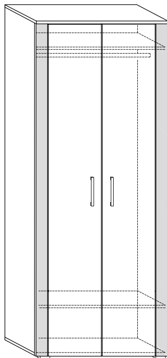
NOT-07 SZAFKA H-205 D-56 L-80
