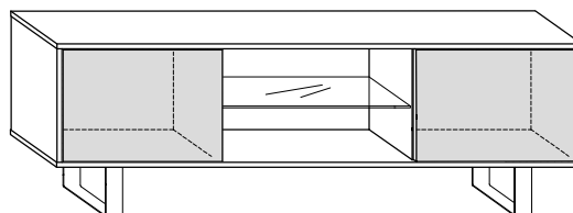
H-53 D-36 L-160 KIN-02 STOLIK RTV DUŻY
