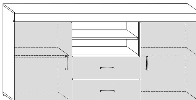
H-80 D-47 L-164 MAM-01 KOMODA
