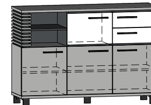
LAM-04 Komoda 4D2S L-135 H-94 D-42
