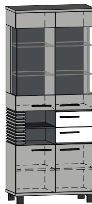
LAM-15 Witryna W2D2S L-80 H-190 D-42
