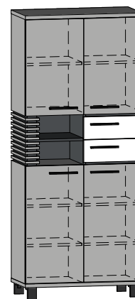
LAM-09 Regał W4D2S L-80 H-190 D-42
