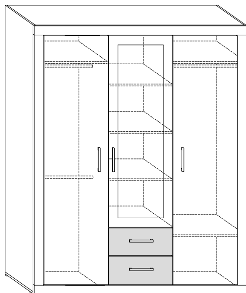
H-209 D-58 L-165 VIK-07 GARDEROBA 3D
