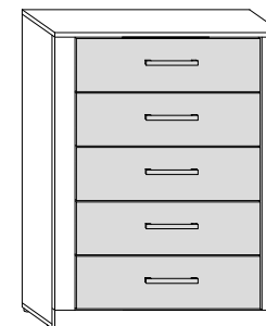
H-106 D-42 L-80 VIK-08 KOMODA MAŁA
